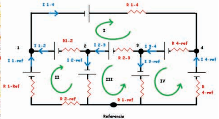
Fig1: Un ejemplo de modelado de la densidad del tráfico en una red viaria utilizando circuitos eléctricos
